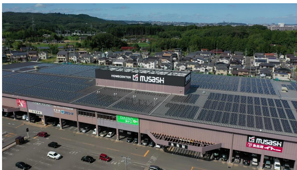
ホームセンタームサシ名取店に設置した太陽光発電システム
